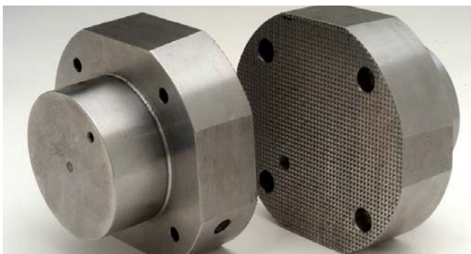
گیره نگه دارنده - تولاکس ۴۴ جایگزین W.Nr. 1.2358 شد، دلیل افزایش طول عمر تا ۴ برابر
