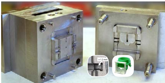
بالا - لیوان پلاستیکی تولید شده با ۱۵٪ هزینه کمتر نسبت به H13/1.2344. پایین - روکش برقی PA6 تولاکس ۴۴ به منظور کاهش زمان ساخت، جایگزین AISI 420 گردید.
